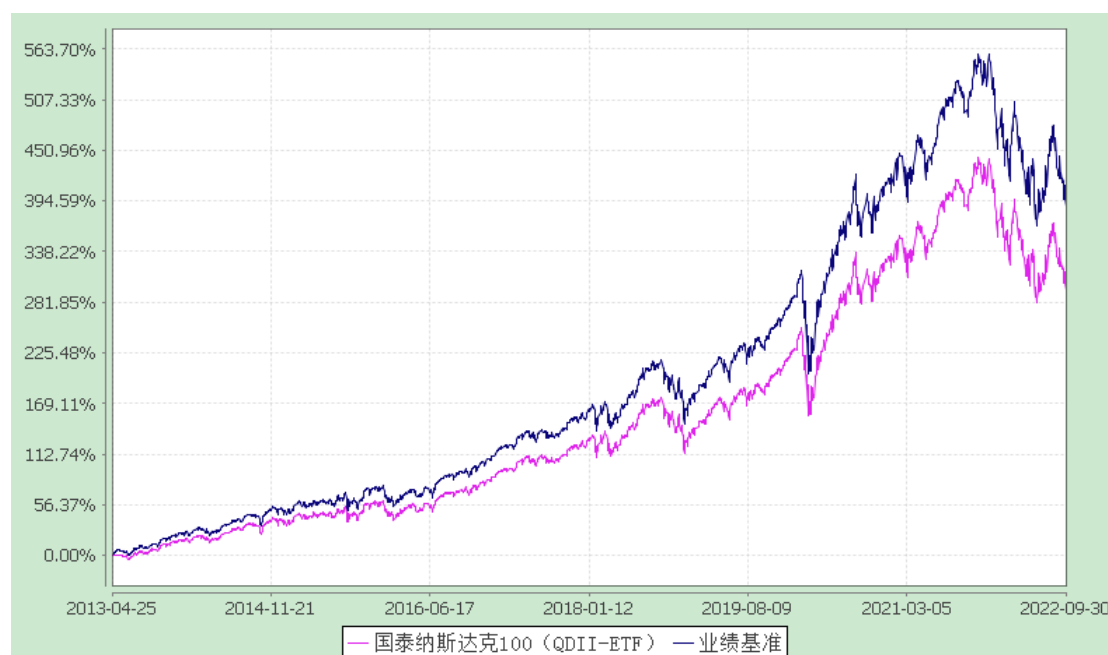
纳斯达克 100 交易型开放式指数证券投资基金 累计净值增长率与业绩比较基准收益率历史走势对比图 (2013 年 4 月 25 日至 2022 年 9 月 30 日)
