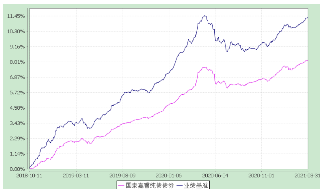
国泰嘉睿纯债债券型证券投资基金 累计净值增长率与业绩比较基准收益率历史走势对比图 (2018 年 10 月 11 日至 2021 年 3 月 31 日)
