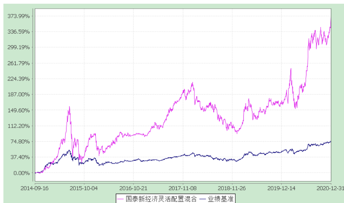
国泰新经济灵活配置混合型证券投资基金 累计净值增长率与业绩比较基准收益率历史走势对比图 (2014 年 9 月 16 日至 2020 年 12 月 31 日)
