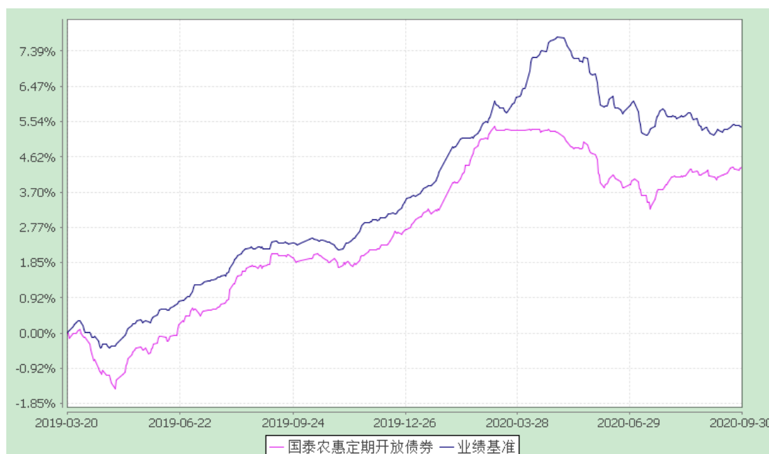
国泰农惠定期开放债券型证券投资基金 累计净值增长率与业绩比较基准收益率历史走势对比图 (2019 年 3 月 20 日至 2020 年 9 月 30 日)
