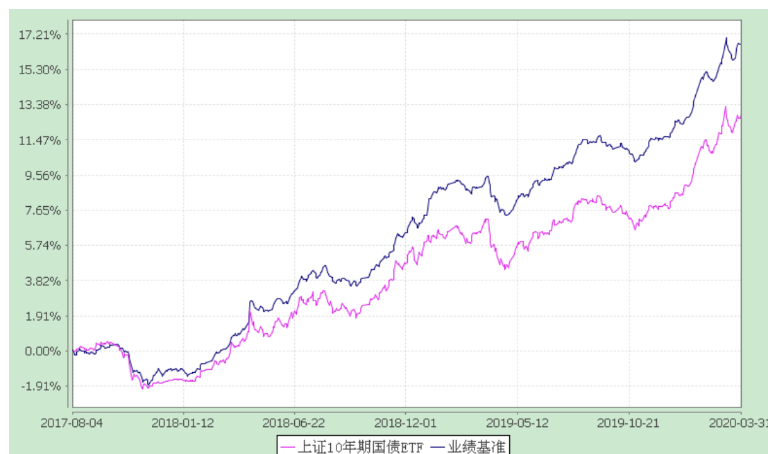
上证 10 年期国债交易型开放式指数证券投资基金 累计净值增长率与业绩比较基准收益率历史走势对比图 (2017 年 8 月 4 日至 2020 年 3 月 31 日)
